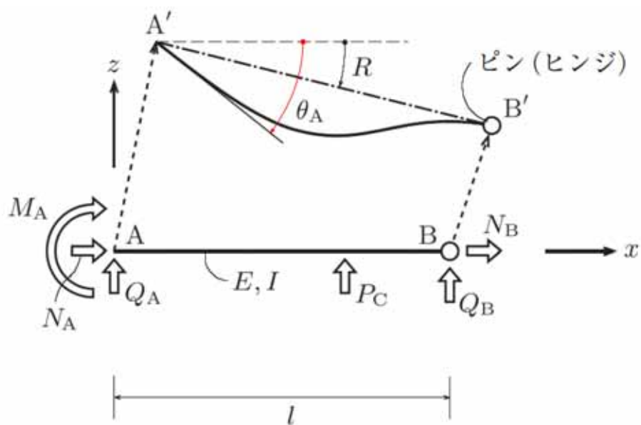
図 6.14 B 点がピン (ヒンジ) 接合された部材 AB に加わる力と変形
