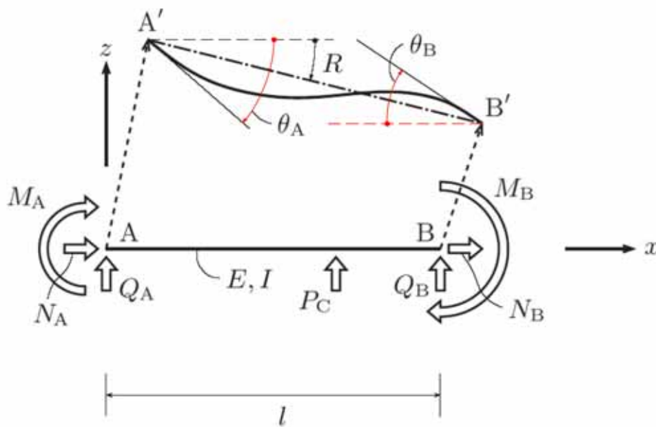
図 6.6 部材 AB に加わる力と変形
